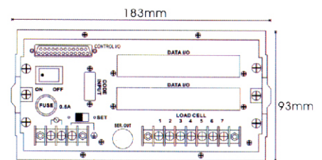
後視圖 Rear View
