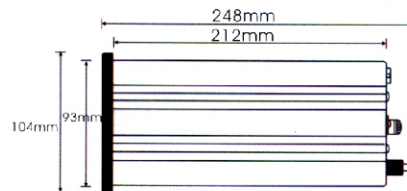
側視圖 Side View
